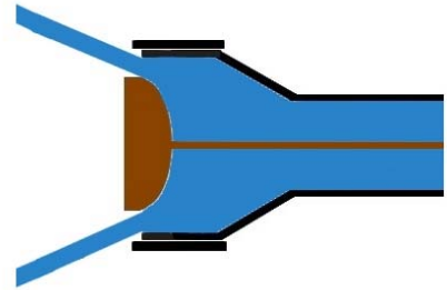
Bild 2: Umlenkkörper am Düsenaustritt erzeugt einen Sprühstrahl (schematische Darstellung) 2 und 3).
